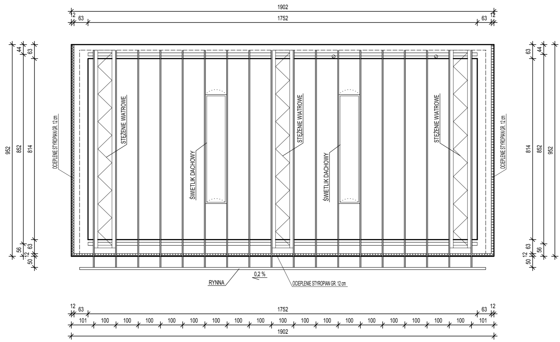
RZUT WIĘZBY DACHU 1:100
