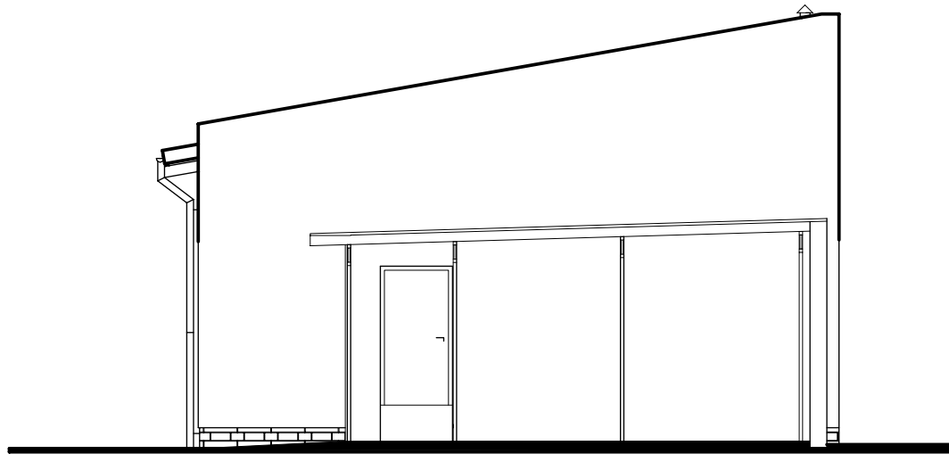
ELEWACJA POŁUDNIOWA 1:100
