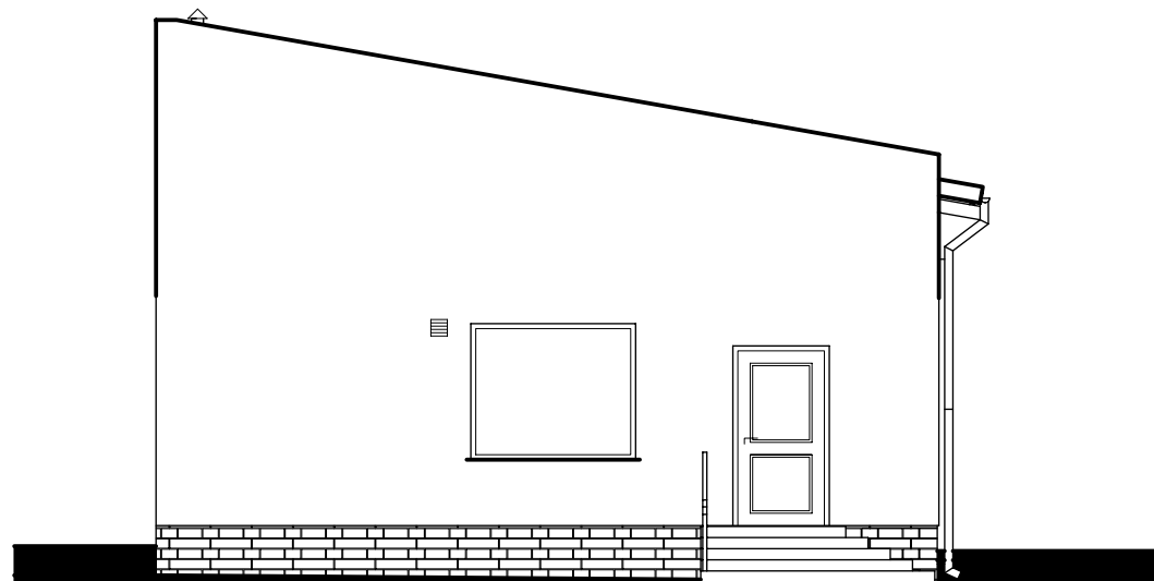
ELEWACJA PÓŁNOCNA 1:100
