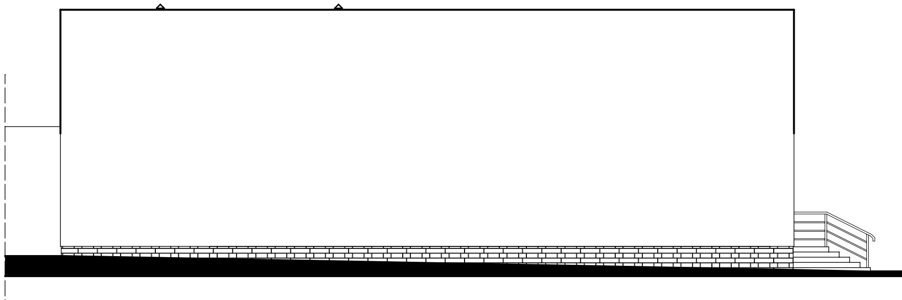
ELEWACJA WSCHODNIA 1:100
