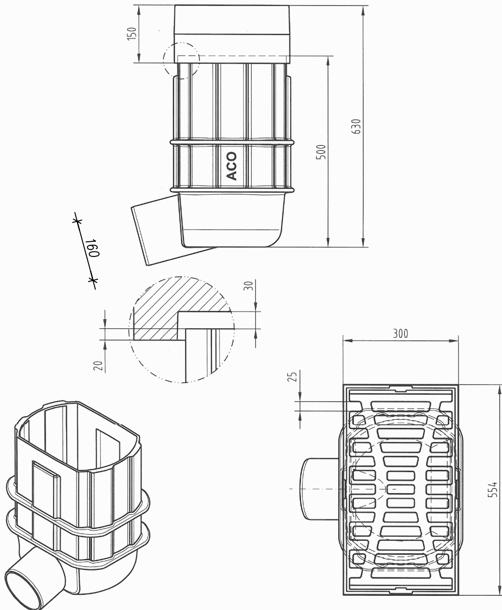
WPUST ULICZNY ACO Combipoint, wesja niska lub równoważny
