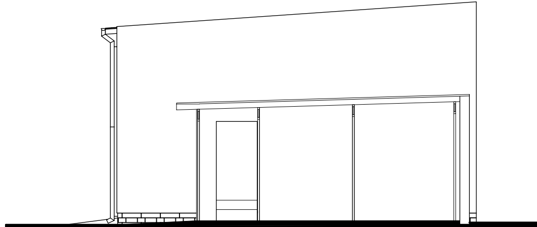
ELEWACJA POŁUDNIOWA 1:100 - INWENTARYZACJA
