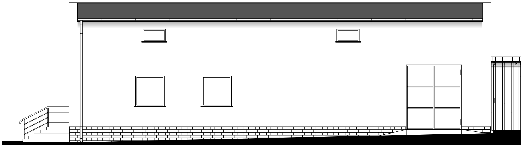
ELEWACJA ZACHODNIA 1:100 - INWENTARYZACJA
