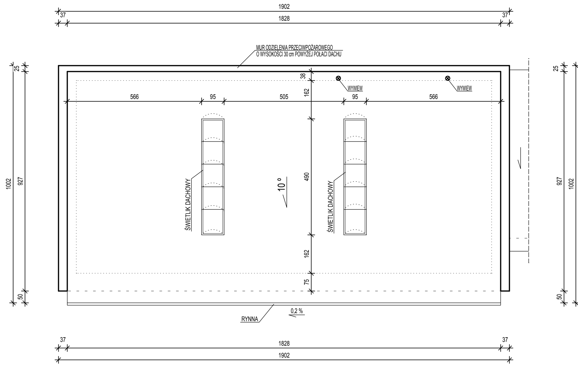
RZUT DACHU 1:100
