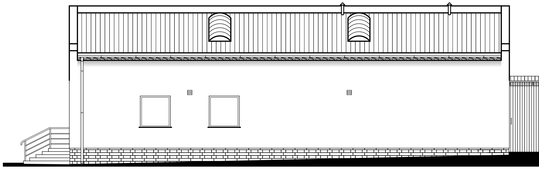
ELEWACJA ZACHODNIA 1:100
