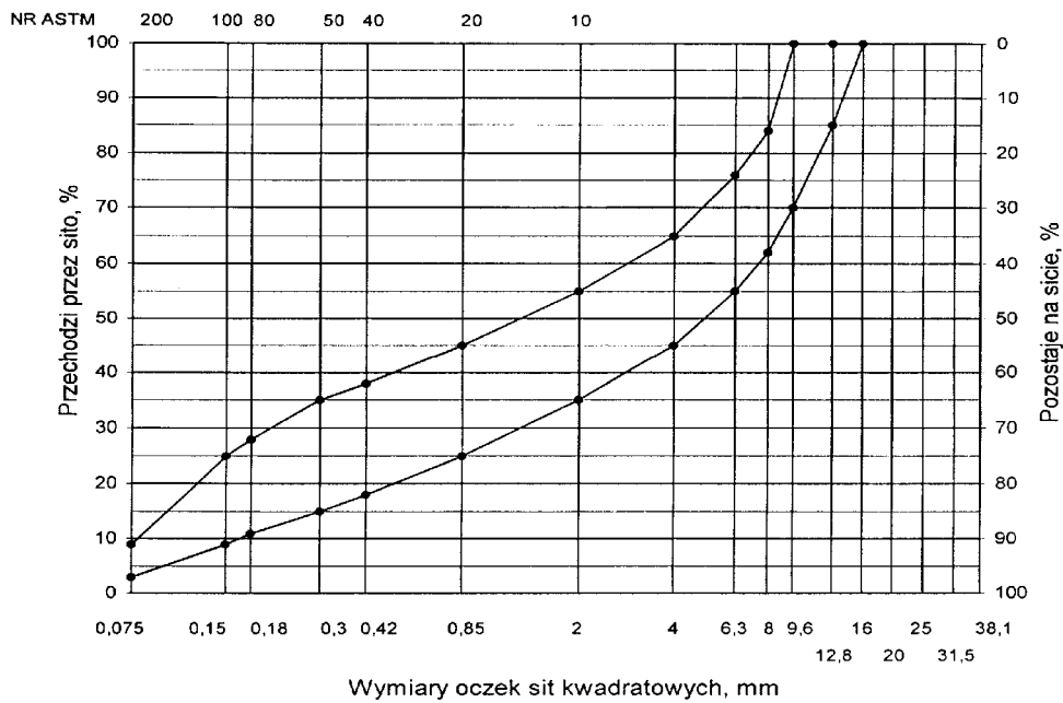
Rys. 10. Krzywe graniczne uziarnienia mieszanki mineralnej BA od 0 do 12,8 mm do warstwy wiążącej, wyrównawczej i wzmocniającej nawierzchni drogi o obciążeniu ruchem KR1 lub KR2
